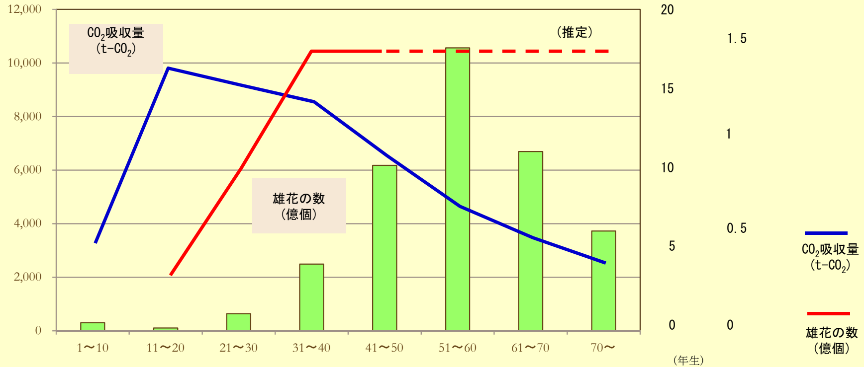
年齢別面積とhaあたりの「スギのCO 2 吸収量」「雄花の数」
