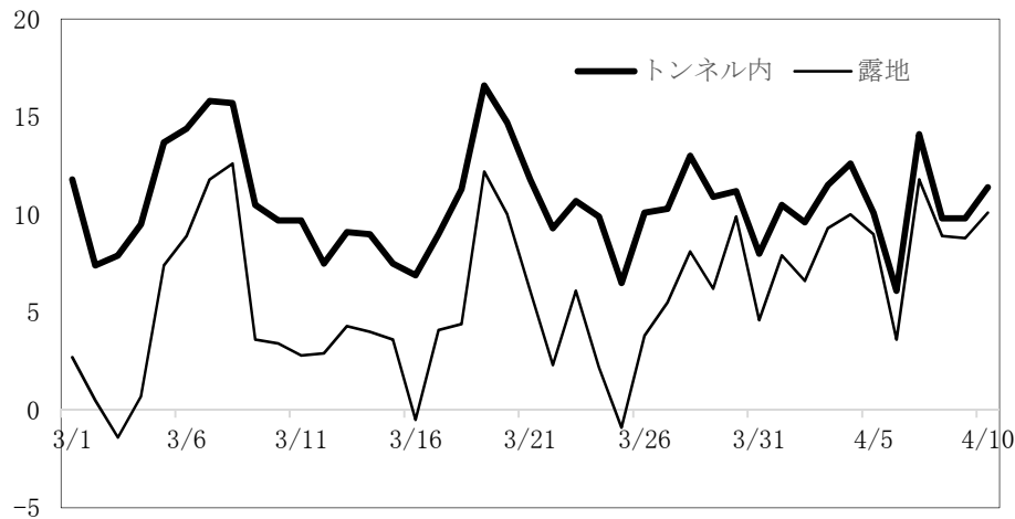
図1 トンネル内と露地の最低気温の推移
