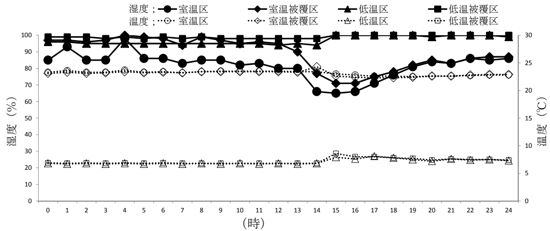
図1 貯蔵6日目（9月21日）における各貯蔵方法の温湿度の推移
