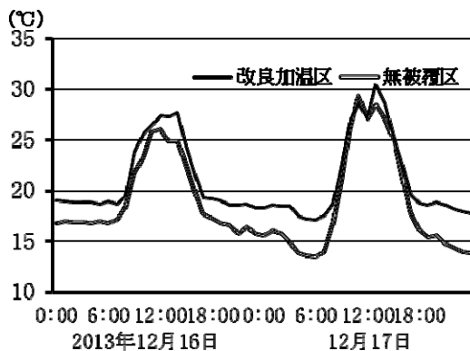
図4 加温装置および自動換気の有無によるハウス内温度の変化
