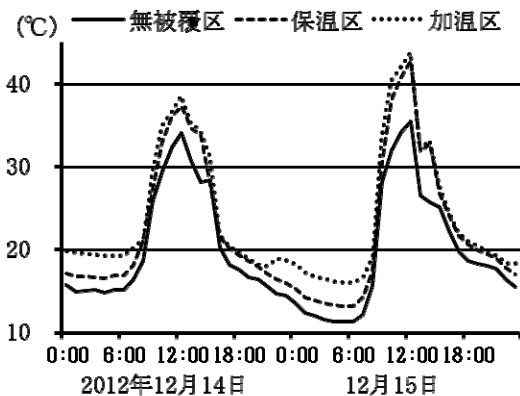
図3 二重被覆および加温装置の設置によるハウス内温度の変化
