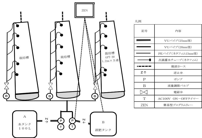
図1 試作した鉢花用点滴灌水装置 (TNS-1 型) (成果 1)
