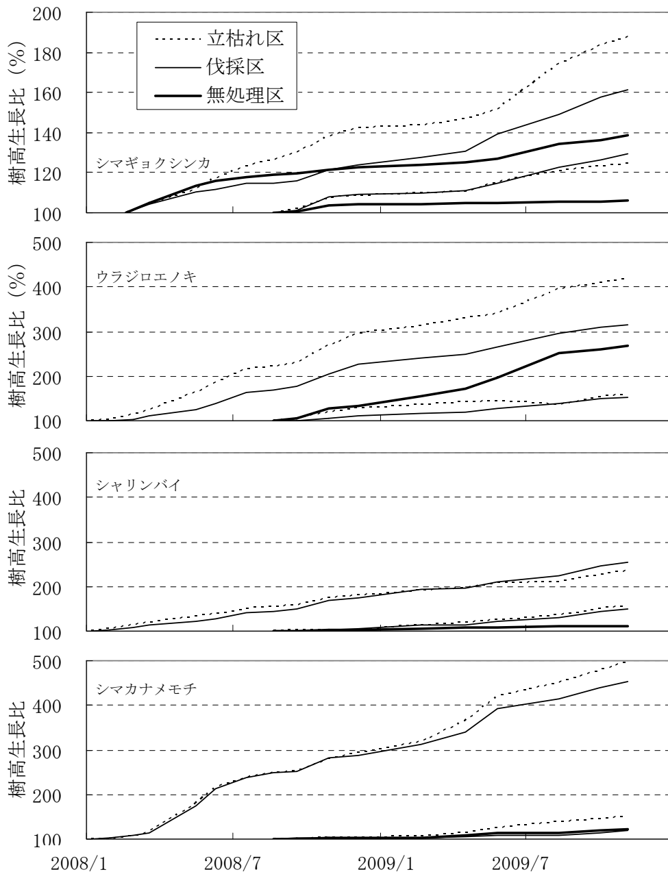
図1 モクマオウ林に移植した固有種および広分布種の樹高生長比
