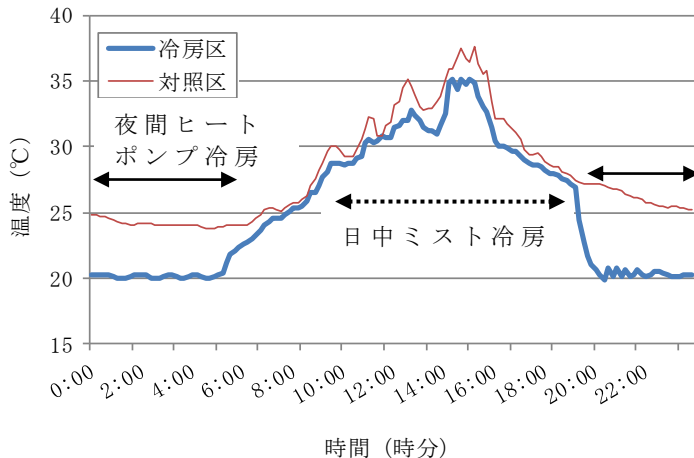
図1 冷房による温度制御 2011年7月27日のデータ
